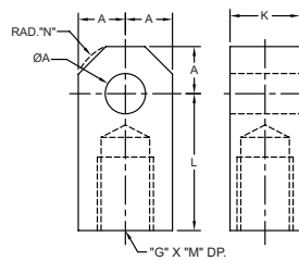
Rod Eye
